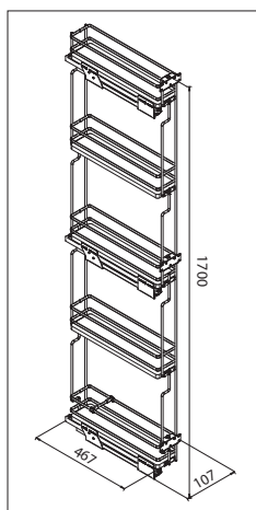
Varijanta s ugradnjom na desno
