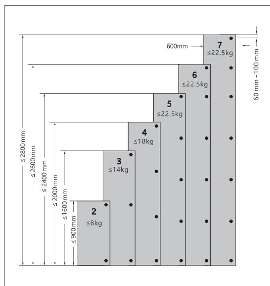
Skica određivanja bušenja.
