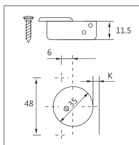
Skica određivanja bušenja.
